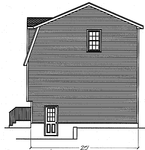
Right Elevation
