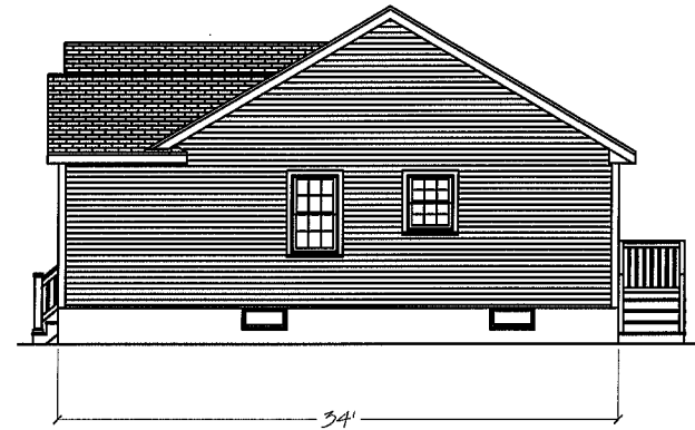
Right Elevation
