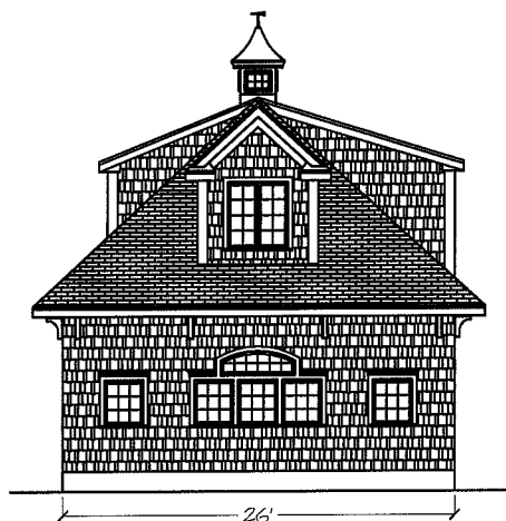
Right Elevation
