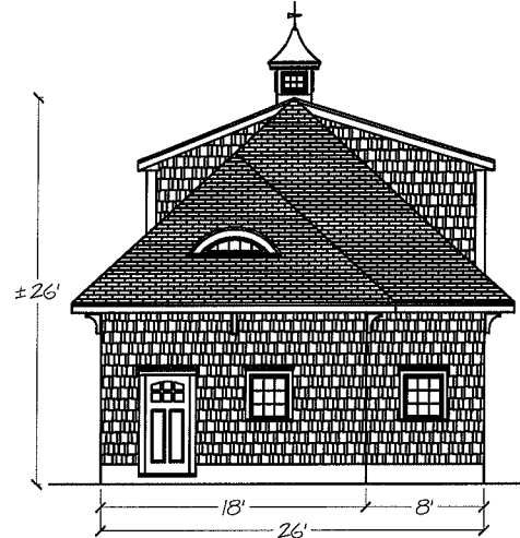
Right Elevation
