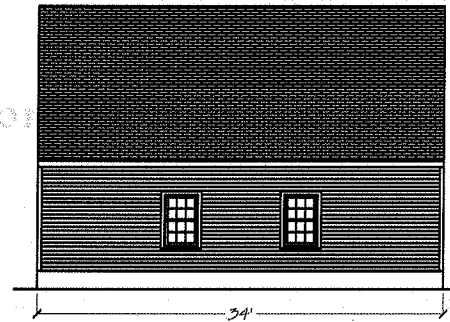
Right Elevation
