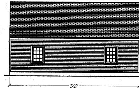
Right Elevation
