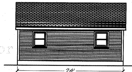
Right Elevation
