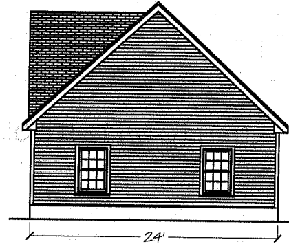
Right Elevation
