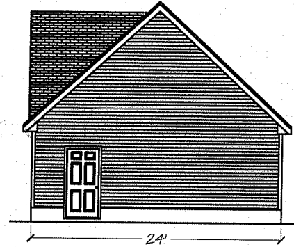
Right Elevation
