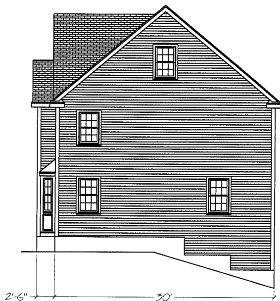
Right Elevation
