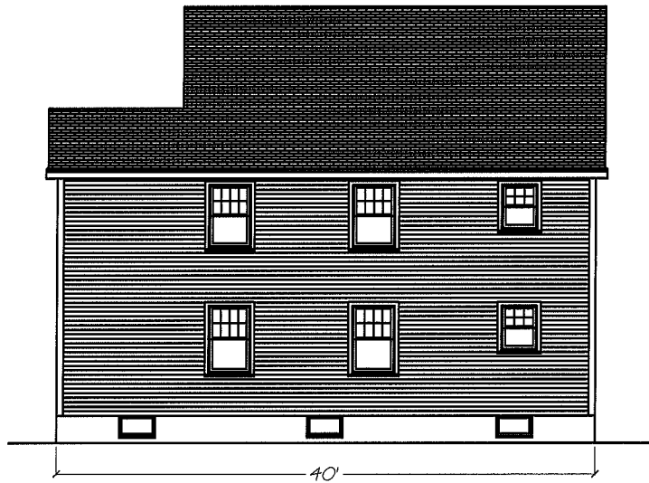
Right Elevation
