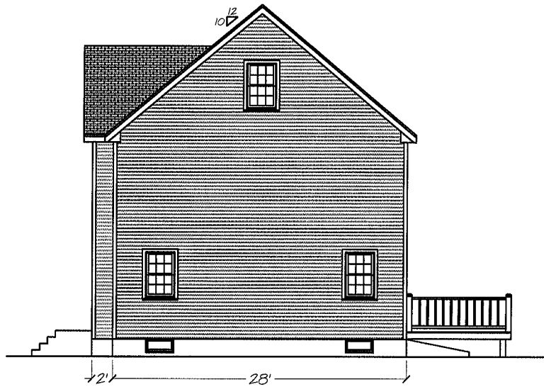
Right Elevation
