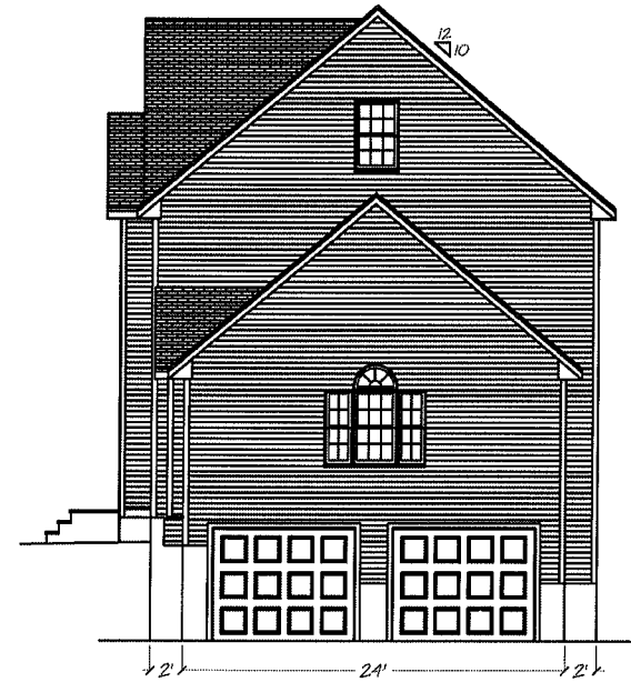
Right Elevation
