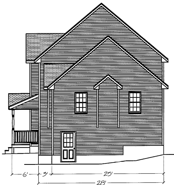
Right Elevation
