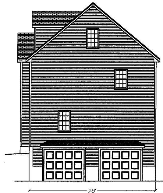
Right Elevation
