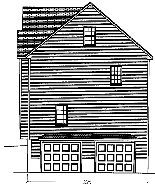
Right Elevation
