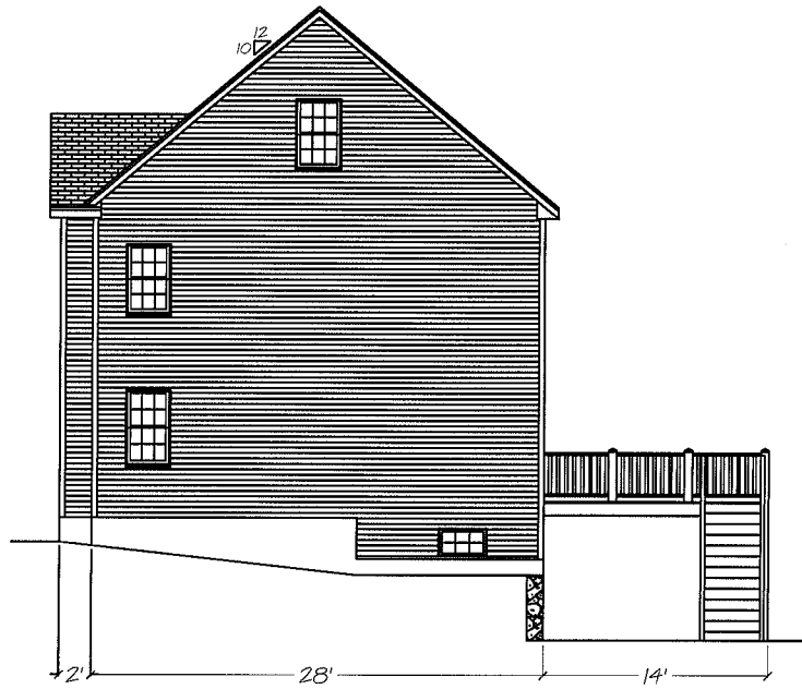
Right Elevation
