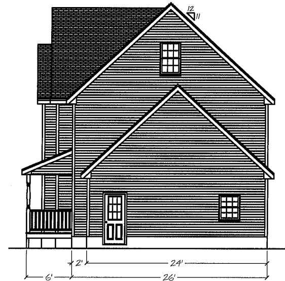
Right Elevation
