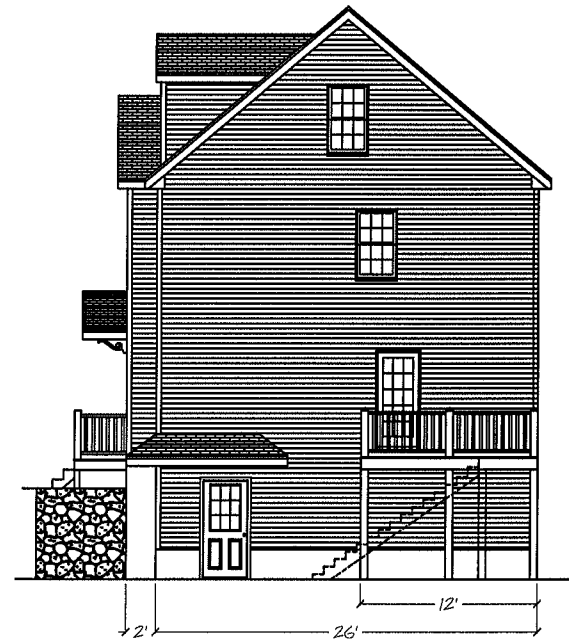
Right Elevation
