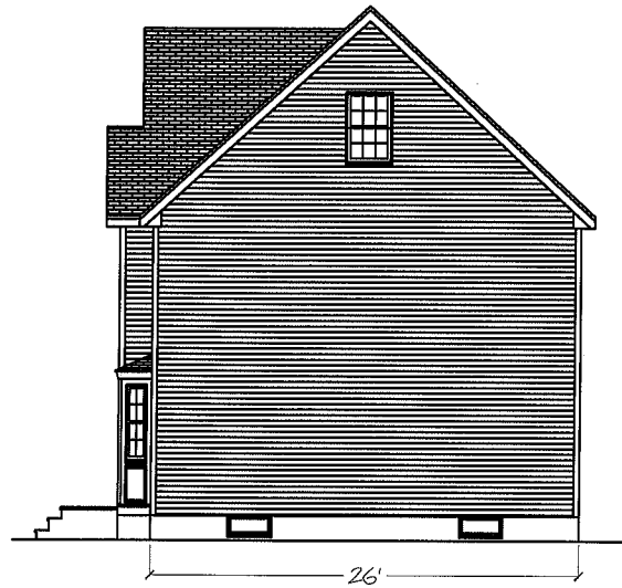
Right Elevation
