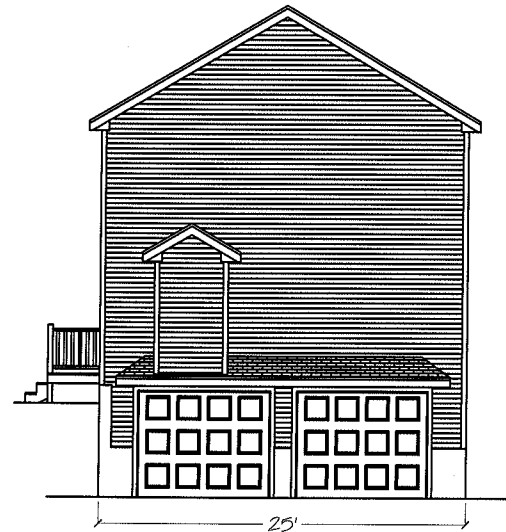
Right Elevation
